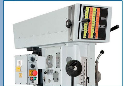
VAR.R (Variatore ritardo) • VAR.R (Variateur par engrenages) • VAR.R (Speed variator with gears) • VAR.R (Stufenlos mit Getriebe)
